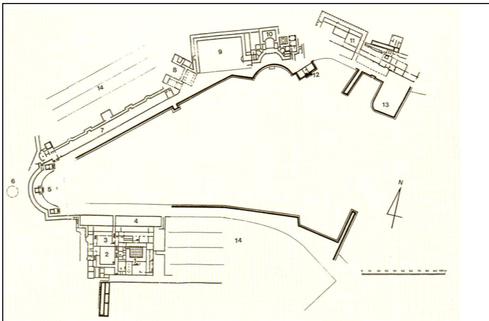
Sl. 156. Ladanjska vila, uvala Verige, o. Veliki Brijun: 1. prvotna villa rustica , jezgra kompleksa; 2. dogradeni peristil; 3. rezidencijalni dio; 4. terase i trijem s lodama; 5. potez hramova s prospektom prema moru; 6. temelj kružnog objekta; 7. temelj portika s kriptoportikom; 8. diaeta ; 9. palaestra ; 10. terme s aneksima; 11. gospodarski dio; 12. bazen za ribe ( vivarium ); 13. antičko pristanište; 14. vrtovi na terasama; Gnirs 1915.; Begović Dvoržak 1998.
