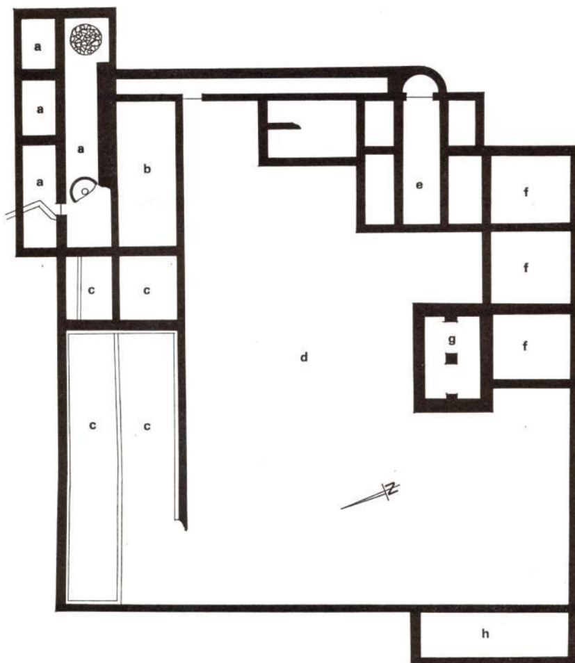
150) Rustička vila u Velikoj Šaraji kod Pule, tlocrt: a — periferni trakt za mljevenje i tiještenje maslina; b — spremište za prikupljanje masline prije obrade; c — spremište za ulje; d — središnje dvorište; e — boravište rustičke familije s kuhinjom i spremištem; f — spremište za alat, pribor i sl.; g — cisterna za sakupljanje kišnice s potpornjacima; h — vjerojatno spremište ili staja (Mlakar).
